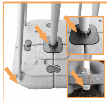
Do připraveného podstavce vsuňte teleskopickou konstrukci a použijte zabezpečovací prvky.
