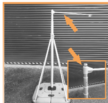
Na horní část konstrukce připevněte kolmé ráhno a zajistěte šroubem.
